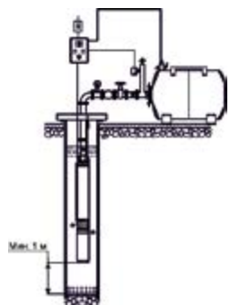
С накопительным резервуаром (гидроаккумулятором) или цистерной.
