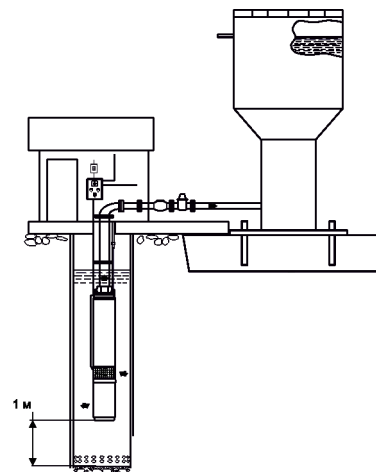
С водонапорной башней Рожновского.
